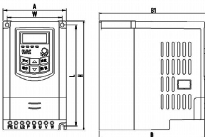
Obudowa plastikowa
