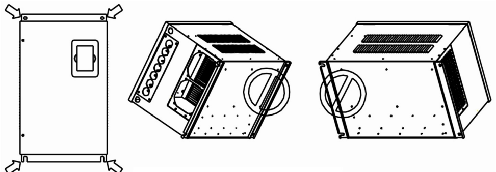
Instalacja w pionie
