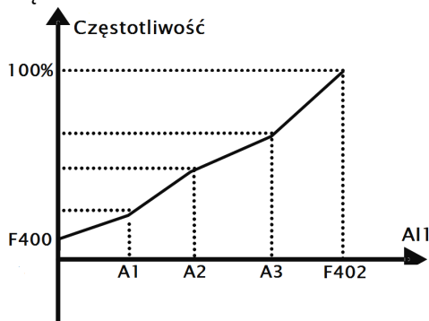
Zależność częstotliwości od wartości sygnału analogowego AI1
