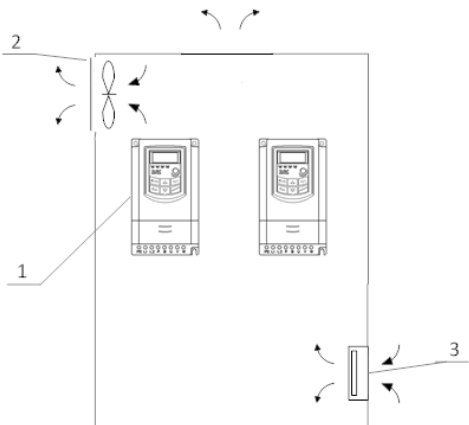
Montaż prawidłowy
