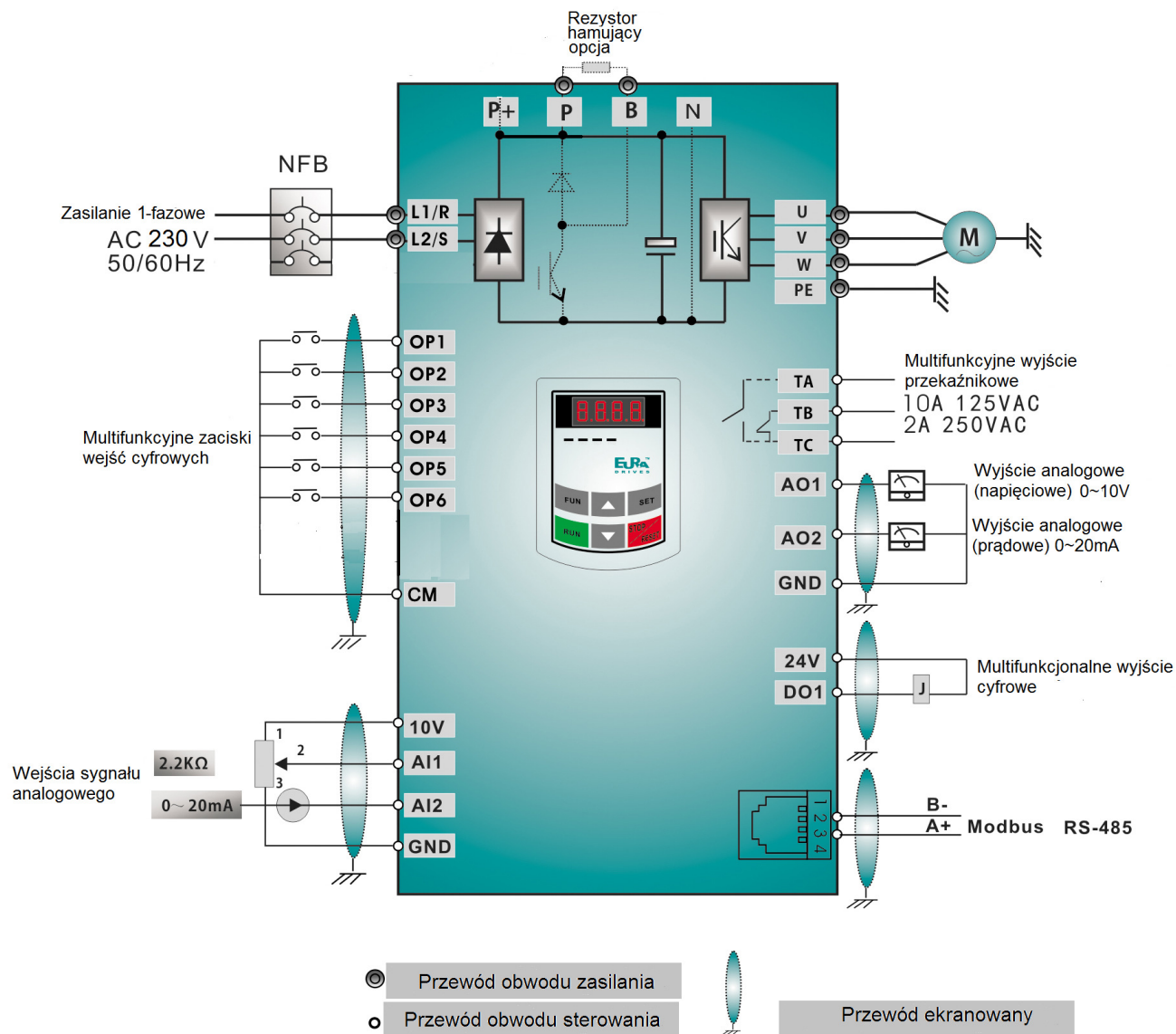
Standardowy układ połączeń przemiennika 1-fazowego (polaryzacja NPN)
