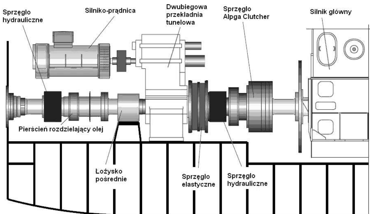
Rys. 5.4 Pomocniczy układ napędowy firmy MAN B&W
